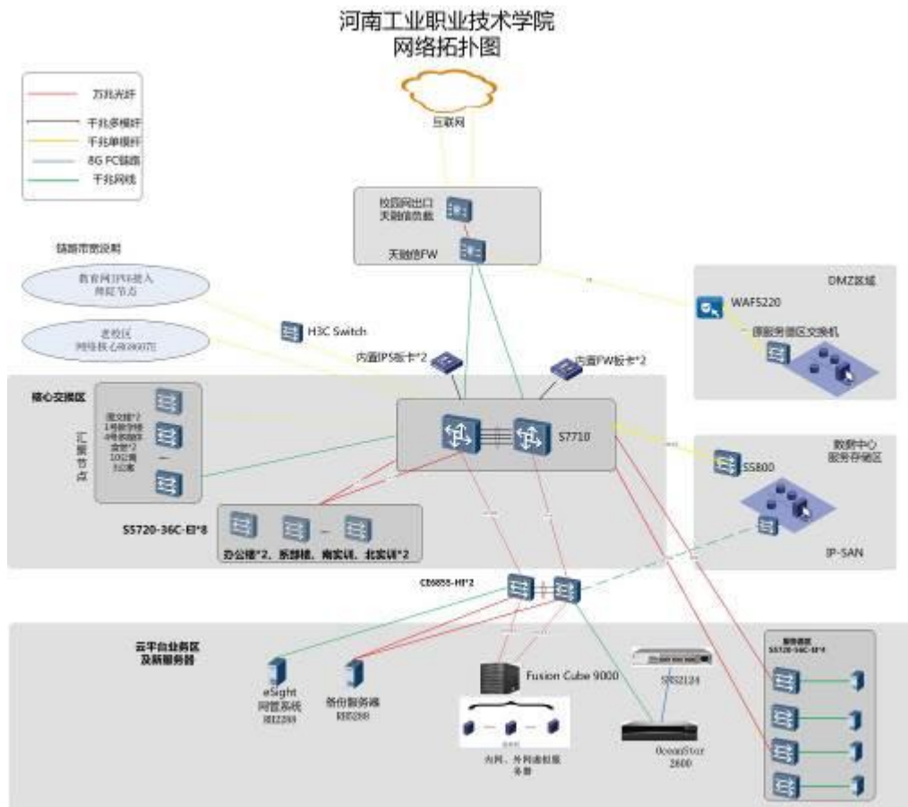
图 1-3 校园网络拓扑图
